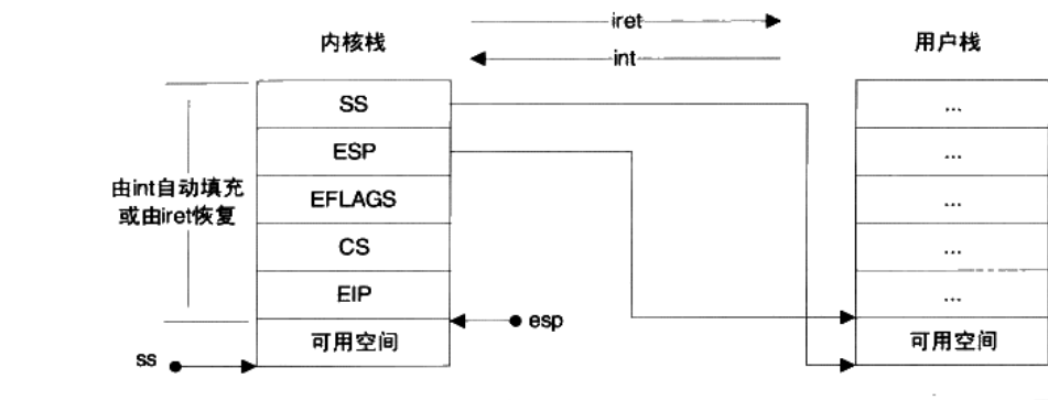
图 12-4 中断时用户栈和内核栈切换
