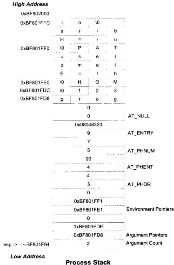
图 7-11 进程初始化堆栈
