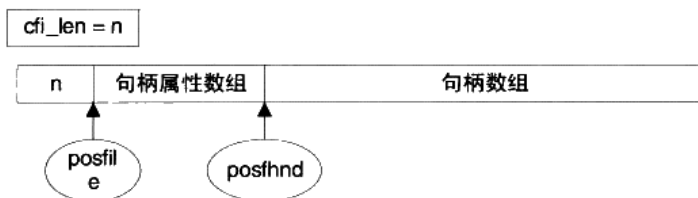
图 11-6 句柄属性数组和句柄数组
