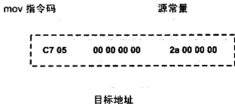
图 2-9 传送指令
