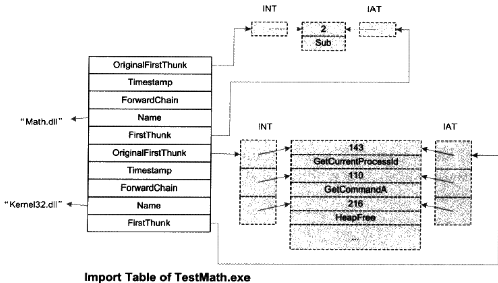
图 9-4 TestMath.exe 导入表
