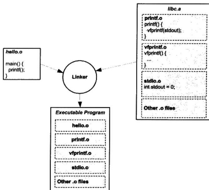
图 4-6 静态库链接
