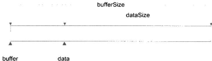
图 11-12 data、buffer、bufferSize 和 dataSize
