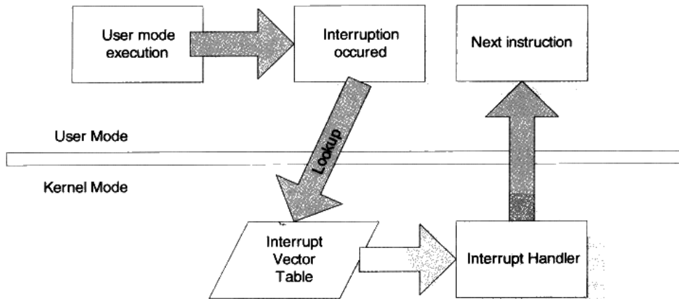
图 12-2 CPU 中断过程
