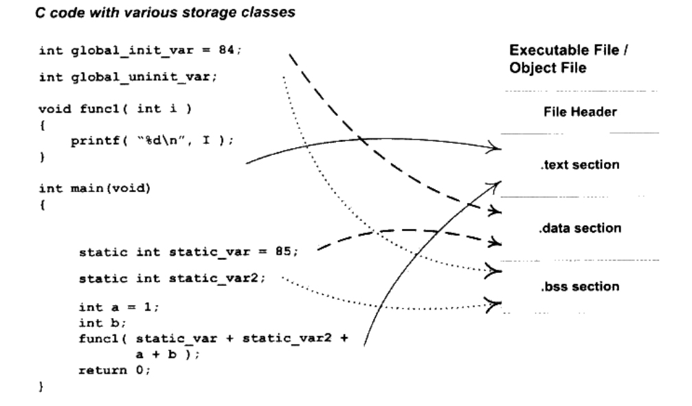
图 3-1 程序与目标文件
