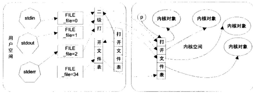
图 11-5 Windows 的 FILE、句柄和内核对象
