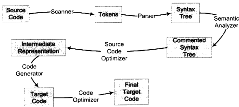
图 2-2 编译过程
