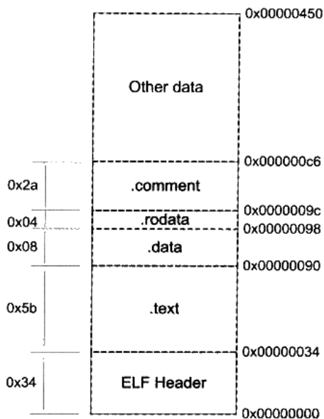
图 3-3 SimpleSection.o
