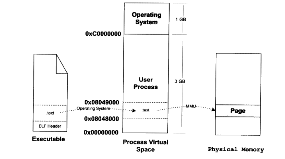
图 6-6 页错误
