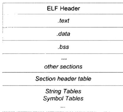
图 3-4 ELF 结构
