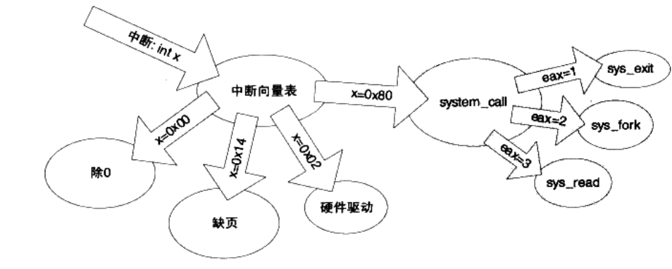
图 12-5 Linux i386 中断服务流程
